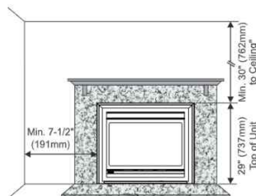
Clearances for Vignette Faceplate
