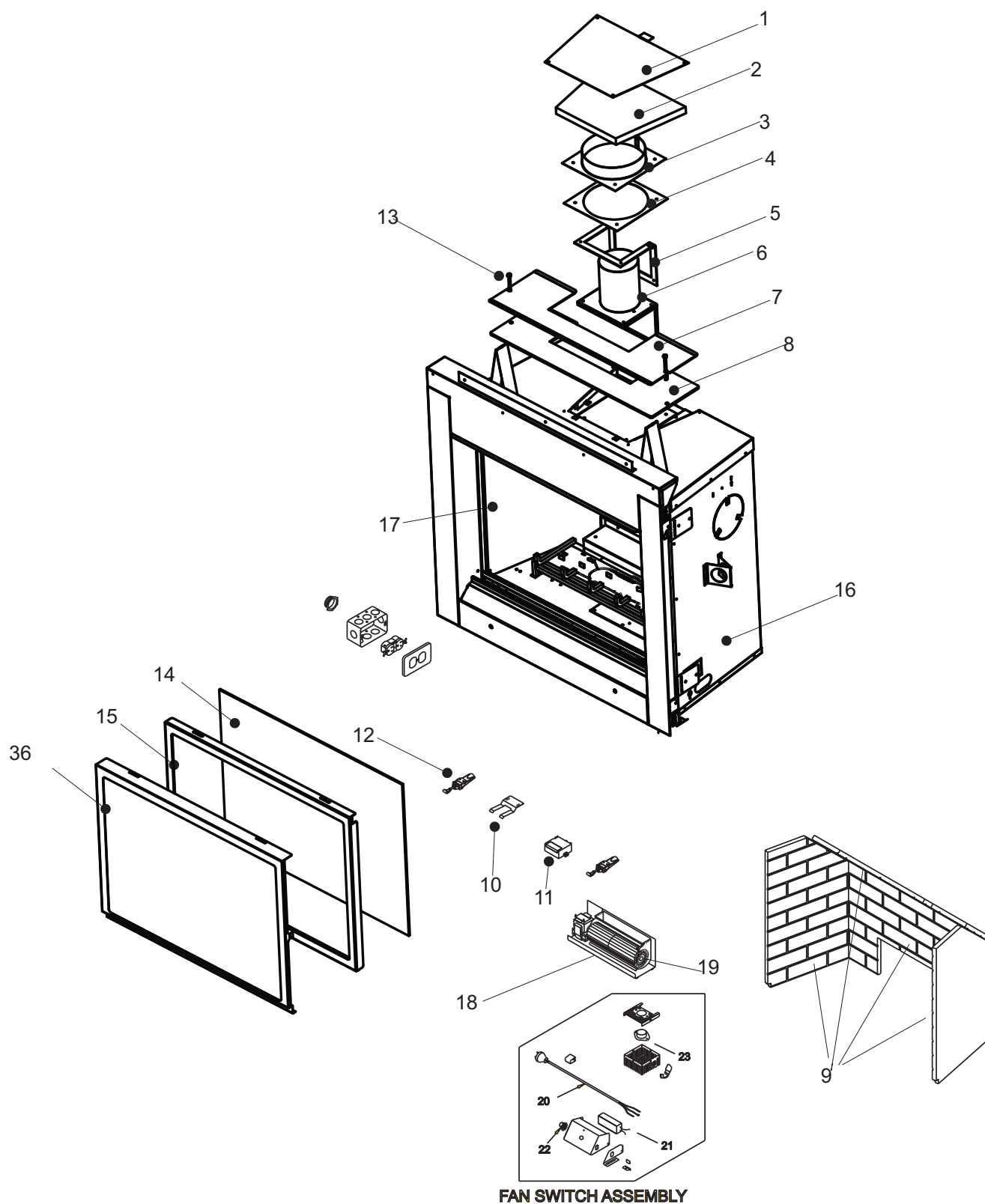
FAN SWITCH ASSEMBLY
